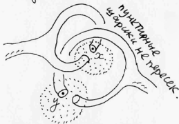
Рис.: Корректность
