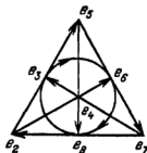
Рис.: Закон умножения в алгебре Oct.K примеру, e_2 e_3 = e_5 .
