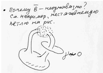
Рис.: Пример петли
