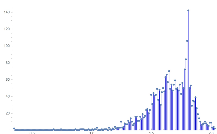
Рис. 17: Распределение количеств пар атомов из разных аминокислот, не связанных ковалентно, по расстояниям между этими атомами.
