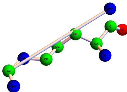
Рис. 9: Файл 1W5Q, 2004 год, RESOLUTION = 1.4.
