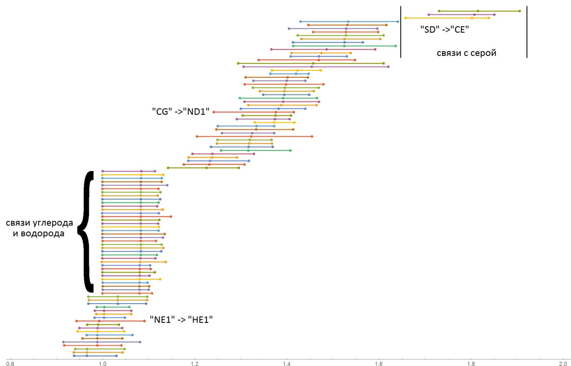
Рис. 10: Распределение интервалов длин ковалентных связей.
