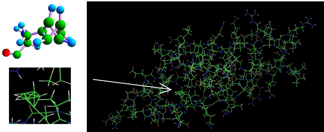
Рис. 3: Файл 2NPL.pdb, 2006 год.
