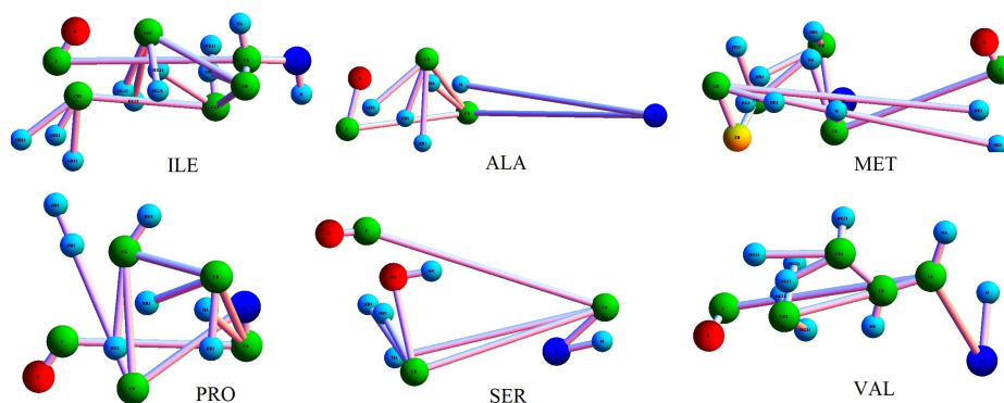
Рис. 1: Некоторые “аминокислоты” из файла 2PDE.pdb (1992 год).
