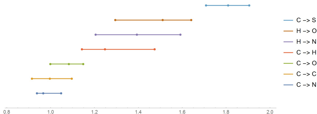
Рис. 19: Интервалы значений разных типов ковалентных связей.
