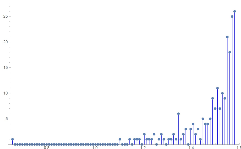
Рис. 16: Распределение количеств пар атомов из одной аминокислоты, не связанных ковалентно, по расстояниям между этими атомами.
