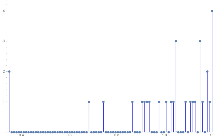
Рис. 18: Распределение количеств пар атомов из разных аминокислот, не связанных ковалентно, по расстояниям между этими атомами.
