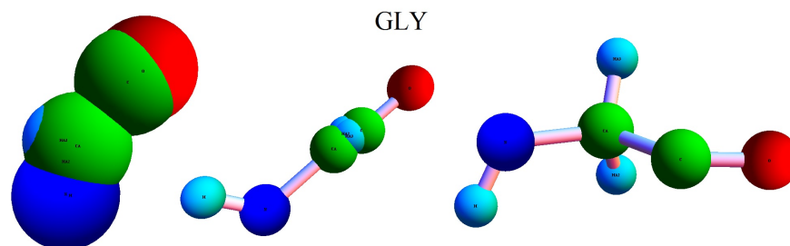
Рис. 2: Слева: два “глицина” из файла 2I2J.pdb (2006 год). Справа — “стандартный” глицин.
