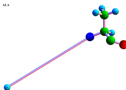
Рис. 4: Файл 2L5R.pdb, 4-ая модель, 19-ая аминокислота, 2010 год, список программ: TOPSPIN 2.0, SPARKY 3.114, CYANA2.0.
