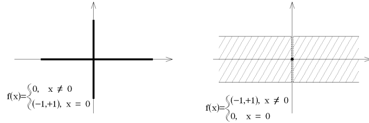
Рис. 3. Многозначное отображение, приведенное на рисунке слева, полунепрерывно сверху в точке 0, но не полунепрерывно снизу; многозначное отображение, приведенное на рисунке справа, полунепрерывно снизу в точке 0, но не полунепрерывно сверху
