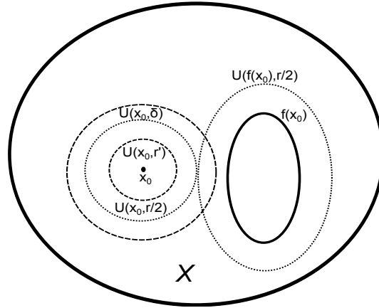
Рис. 4. Иллюстрация к доказательству теоремы Какутани
