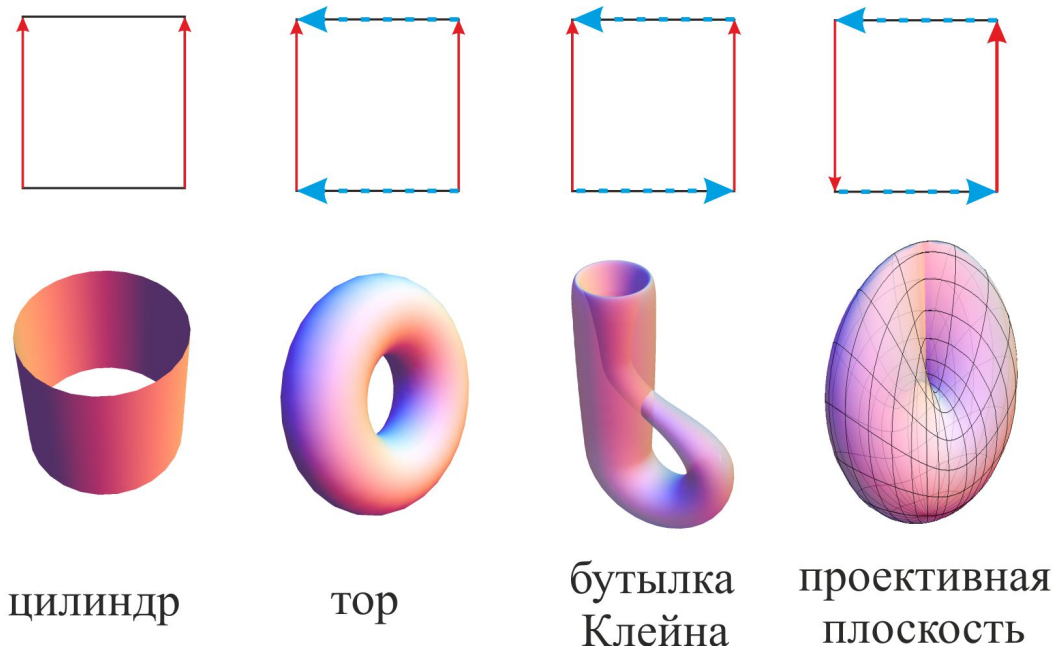
Рис. 12.6: Склейки из квадрата
