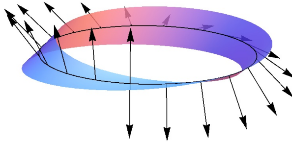
Рис. 12.5: При перемещении нормали к листу Мебиуса вдоль средней линии направление нормали меняется на противоположное.
