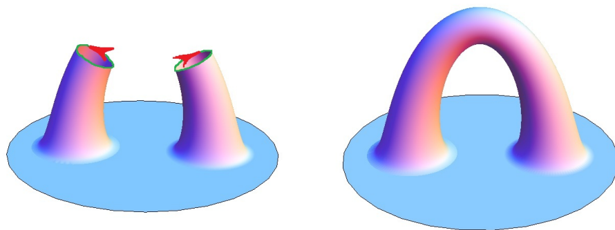
Рис. 12.14: Доказательство теоремы 12.36, шаг 7.
