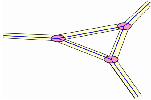
Рис. 12.8: Доказательство теоремы 12.36, шаг 1.
