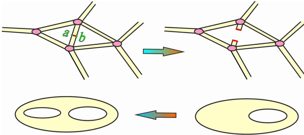
Рис. 12.10: Доказательство теоремы 12.36, шаг 3.
