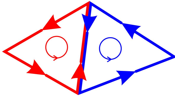
Рис. 12.3: Согласование ориентации симплексов.
