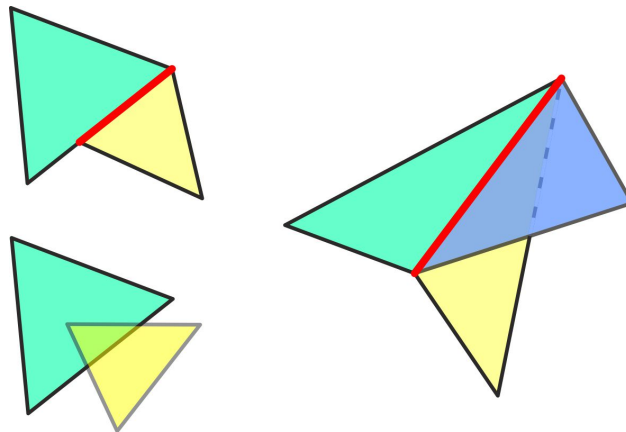
Рис. 12.2: Запрещенные пересечения симплексов.
