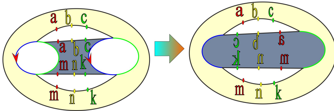
Рис. 12.16: Склейка двух дырок эквивалентна вклейке двух пленок Мебиуса.
