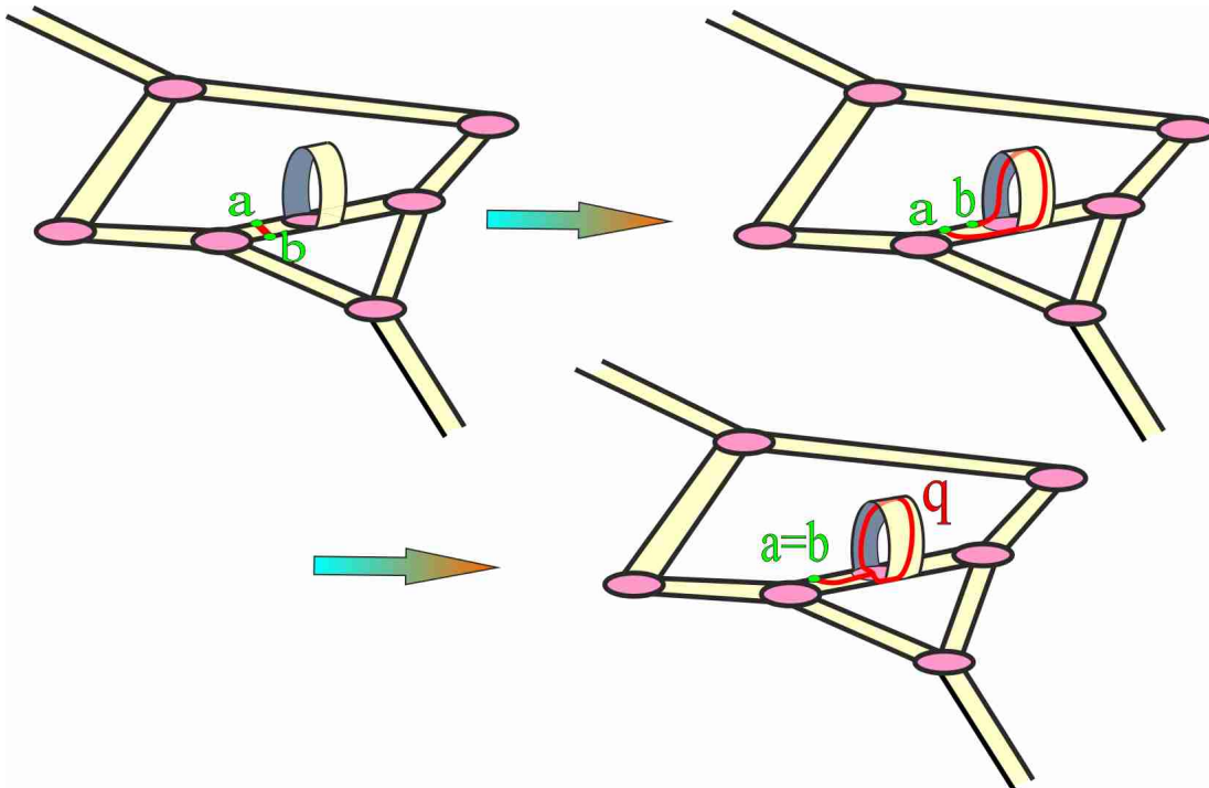
Рис. 12.11: Доказательство теоремы 12.36, шаг 4.
