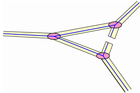
Рис. 12.9: Доказательство теоремы 12.36, шаг 2.
