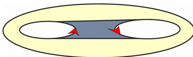
Рис. 12.13: Доказательство теоремы 12.36, шаг 6.
