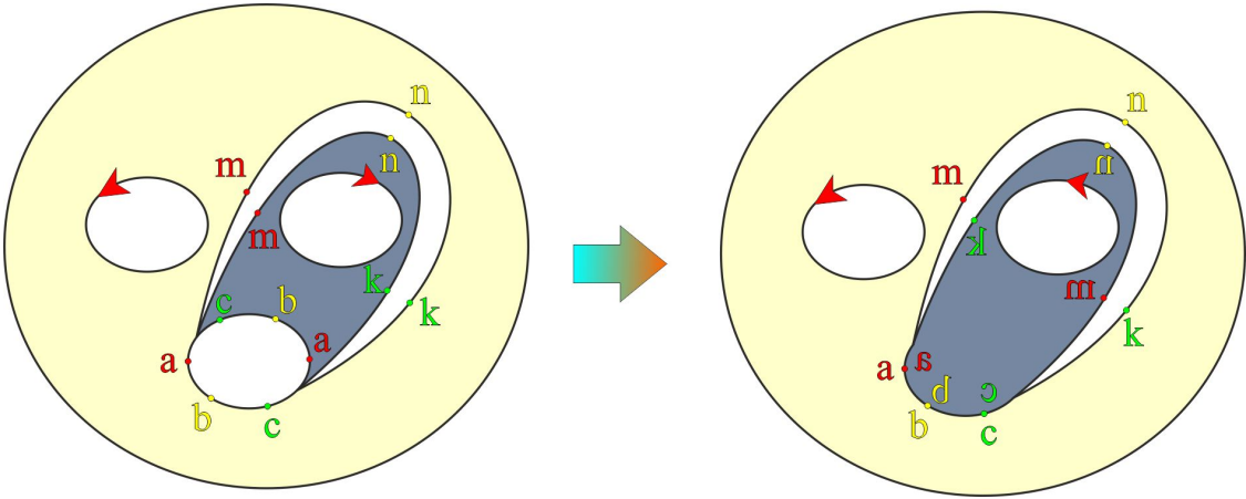
Рис. 12.17: Замена ручки на две пленки Мебиуса.
