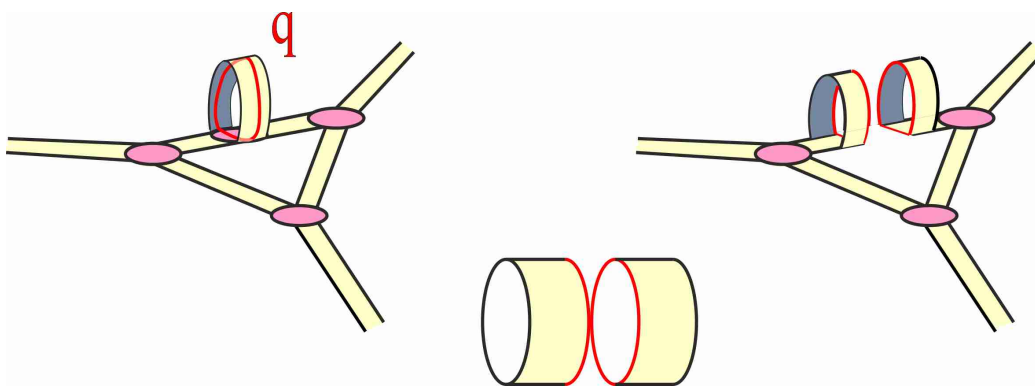
Рис. 12.12: Доказательство теоремы 12.36, шаг 5.
