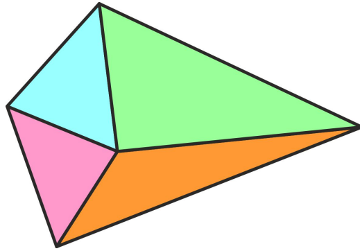
Рис. 12.1: Разрешенное пересечение симплексов.
