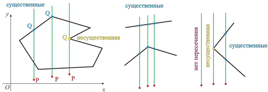
Рис. 3.8: Реализация пункта (3).
