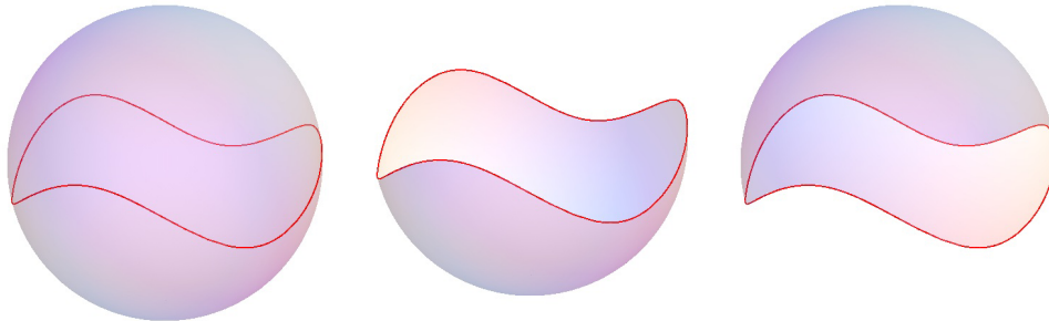
Рис. 3.1: Теорема Жордана верна для сферы.
