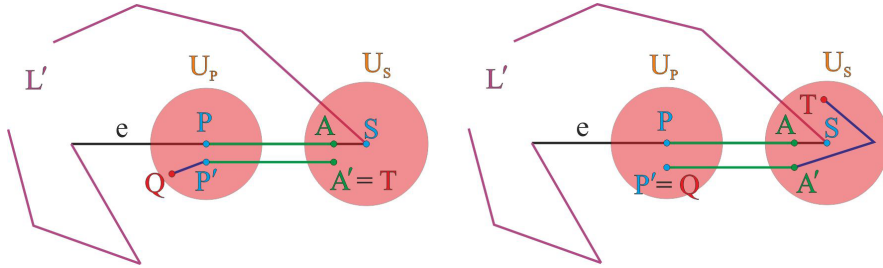
Рис. 3.6: Доказательство леммы 3.18.
