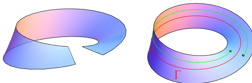
Рис. 3.4: На листе Мёбиуса теорема Жордана не верна.
