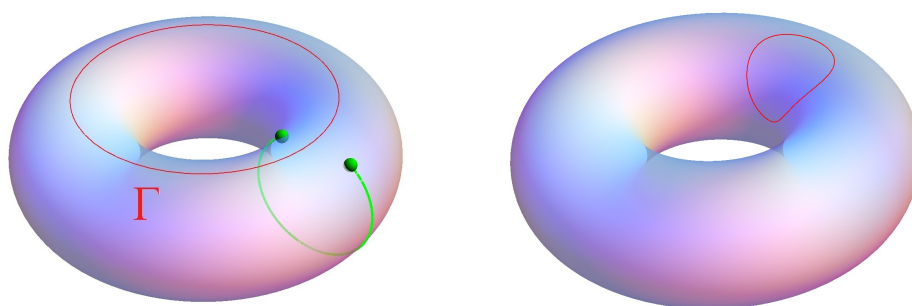
Рис. 3.3: На торе теорема Жордана не верна.
