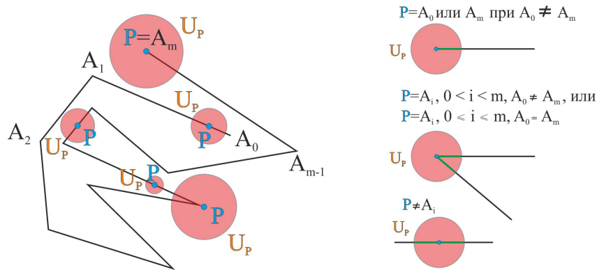
Рис. 3.5: Окрестность U_P .
