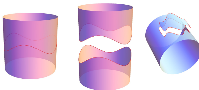
Рис. 3.2: Теорема Жордана верна для цилиндра.
