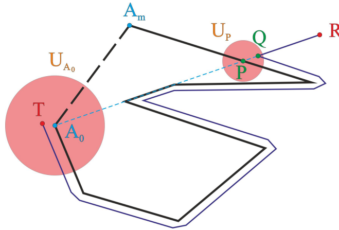
Рис. 3.7: Реализация пункта (3).
